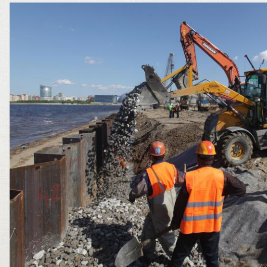
Гидротехнические сооружения
