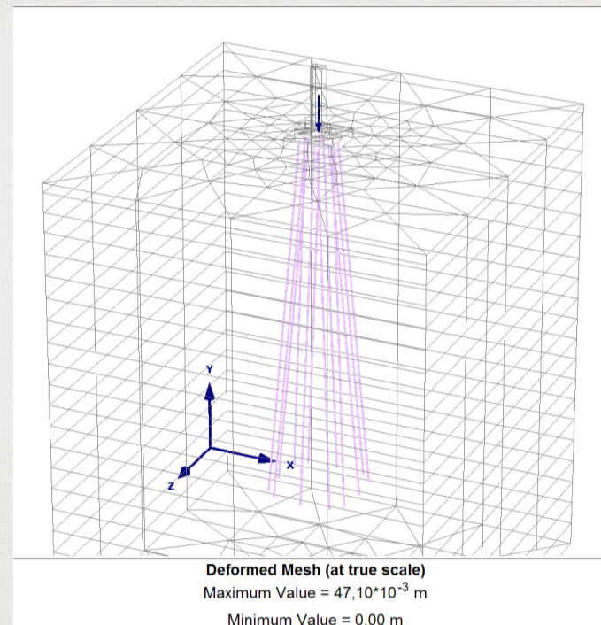
Математическое моделирование куста свай в основании опоры
