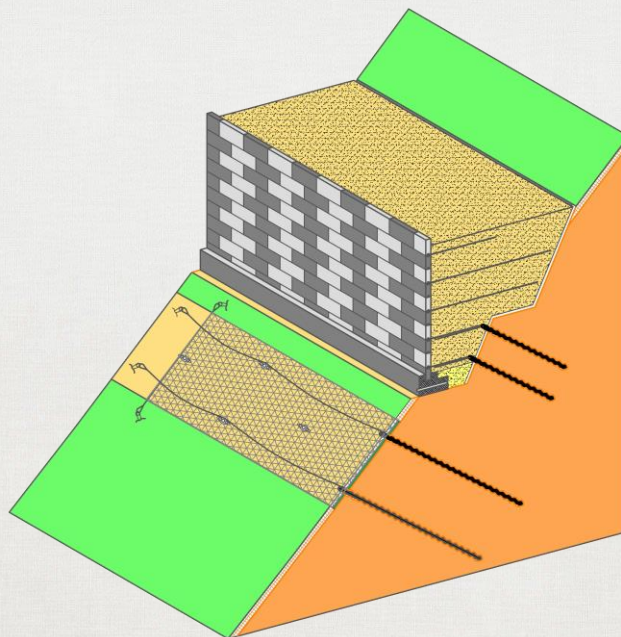
Армогрунтовая система
