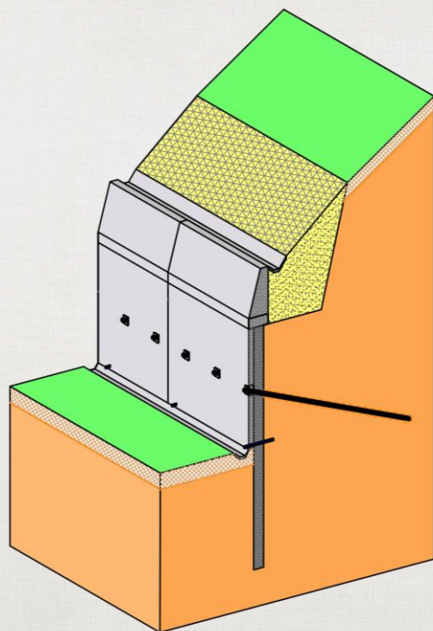
Свайная подпорная стена
