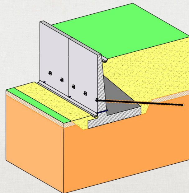
Угловая стена на естественном основании
