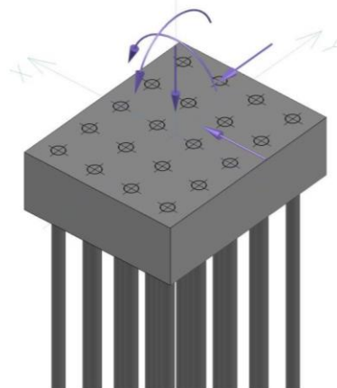
Схема приложения нагрузок на ростверк N12.1, N12.3
