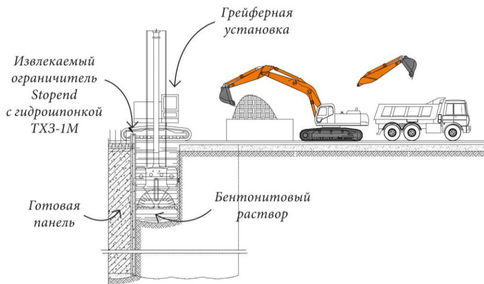
1. Разработка грунта в пределах захватки
