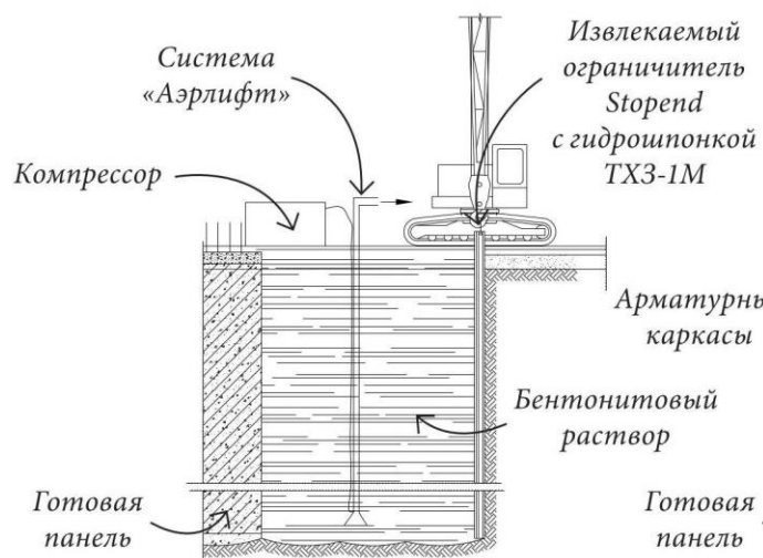
3. Установка ограничителя и десендирование
