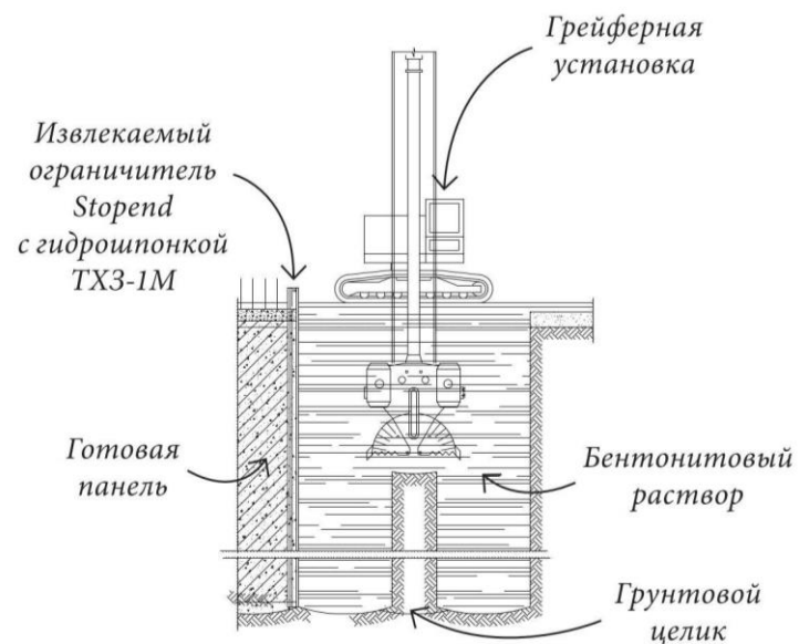
2. Разработка грунтового целика
