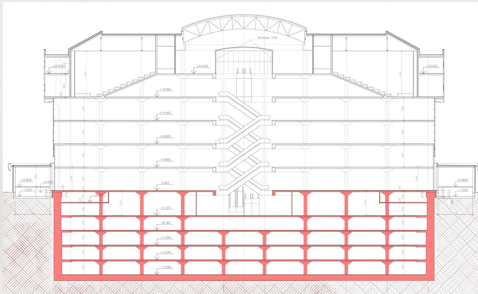
Подземная часть цилиндрической формы диаметром 80 м.
