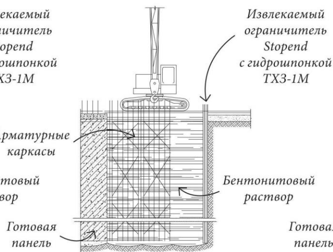
4. Установка арматурных каркасов
