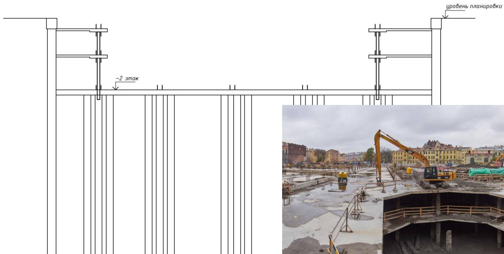
VII этап. Устройство фундаментной плиты.
