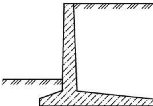
Рисунок Г.2 - Угловая подпорная стена
