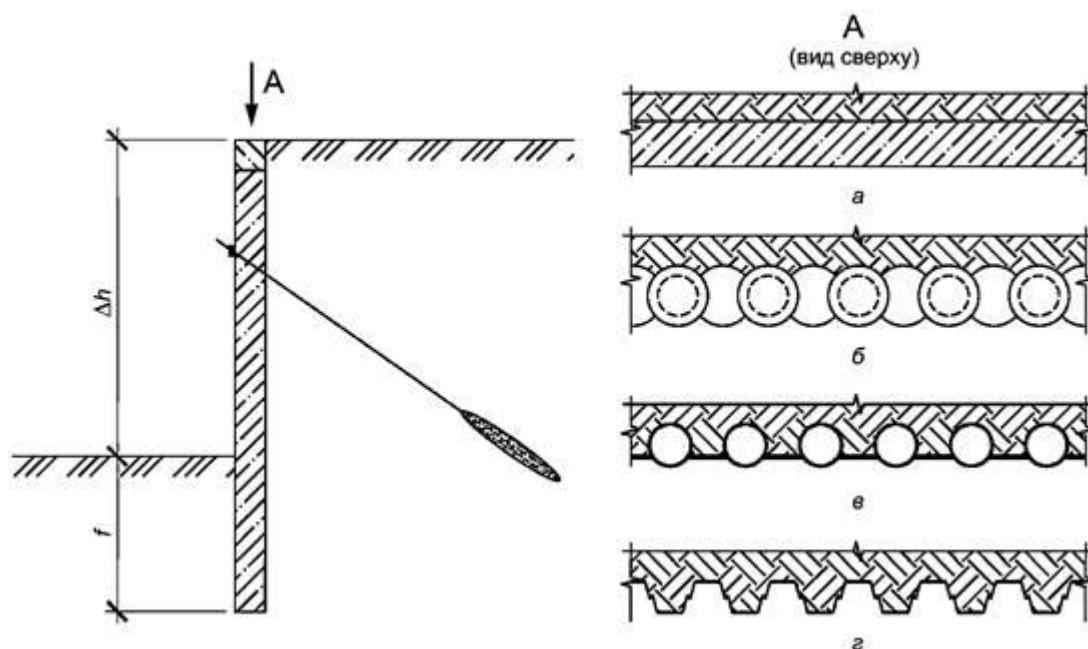
a - траншейная железобетонная «стена в грунте»; б - ограждение из буросекующихся свай; в - ограждение из металлических труб с забиркой; з - шпунтовое ограждение типа «Ларсен»; \Delta h - перепад высот; f - зона заделки
