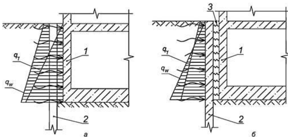
а - водопроницаемое ограждение; б - водонепроницаемое ограждение; 1 - стена подвала; 2 - подпорное сооружение; 3 - упругие связи; p_\gamma - эпюра горизонтального давления от веса грунта и нагрузок на поверхности; q_w - эпюра гидростатического давления воды
