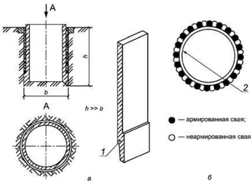
a - колодец (камера) из сборных железобетонных элементов; б - колодец (камера) из буровескующихся свай; 1 - сборный железобетонный элемент; 2 - обвязочный пояс; b - диаметр колодца (камеры); h - высота колодца (камеры), при этом h значительно больше b
