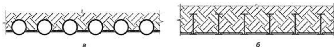
а - ограждение из металлических труб с заборкой; б - ограждение из прокатных профилей
