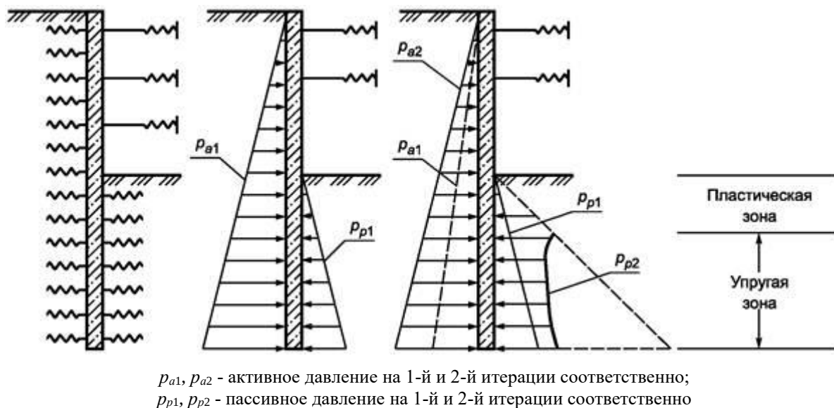
Рисунок 6.9 - Расчетная схема численной контактной итерационной модели гибкого подпорного сооружения
