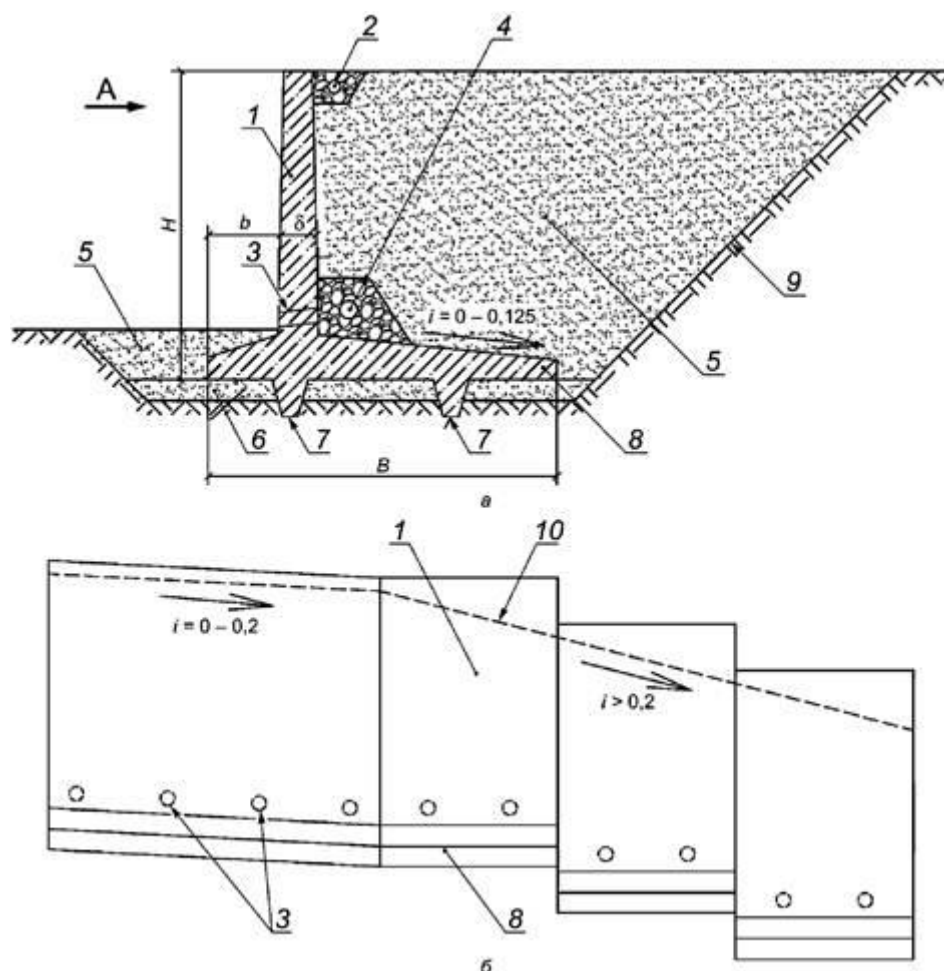
а - поперечное сечение; б - вид спереди (вид А); 1 - лицевая стенка; 2 - водоотводный кювет; 3 - дренажные трубки (шаг - 3 - 6 м); 4 - пристенный дренаж; 5 - обратная засыпка; 6 - подготовка основания «постель»; 7 - «зуб»; 8 - фундаментная плита; 9 - контур траншеи; 10 - контур поверхности земли; i - уклон
