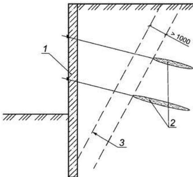
1 - подпорное сооружение; 2 - корень анкера; 3 - теоретическая граница призмы активного давления
