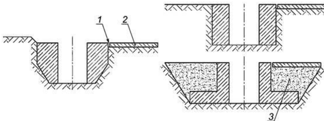
1 - деформационный шов; 2 - технологическая дорога; 3 - обратная засыпка
