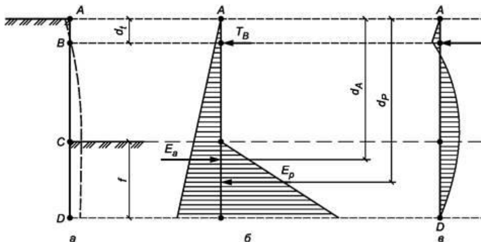
a - деформированная схема конструкции; б - эпюры активного и пассивного давления; в - эпюра изгибающих моментов в стене; d_i - глубина установки яруса крепления; f - искомая глубина заделки;
