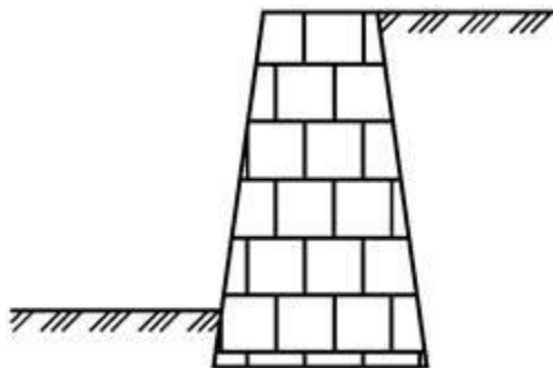
Рисунок Г.1 - Массивная подпорная стена
