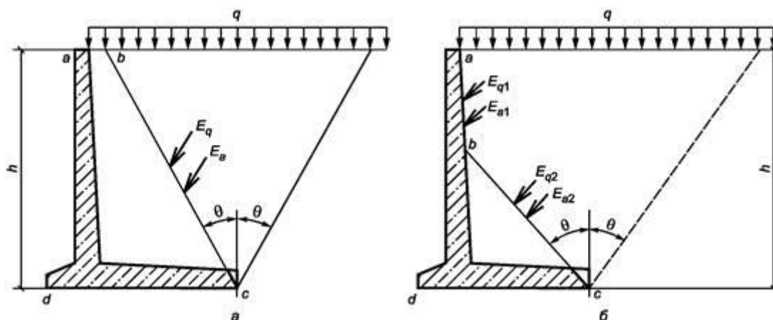
Рисунок 6.6 - Расчетные схемы гравитационных подпорных стен
