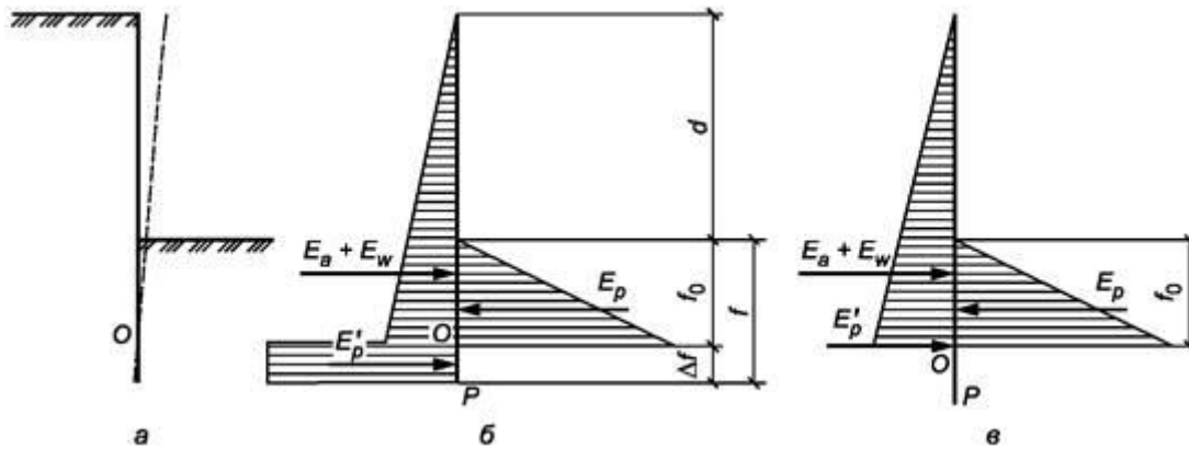
a - деформированная схема; б, в - последовательная аппроксимация активного и пассивного давления; d - глубина котлована; f - заделка стены в грунт; O - точка нулевого момента в стене; P - низ подпорного сооружения; E_a + E_w - равнодействующая активного давления грунта; E_p - равнодействующая пассивного давления грунта; E_w - равнодействующая давления подземных вод; E_p' - равнодействующая противодействия грунта ниже точки нулевого момента
