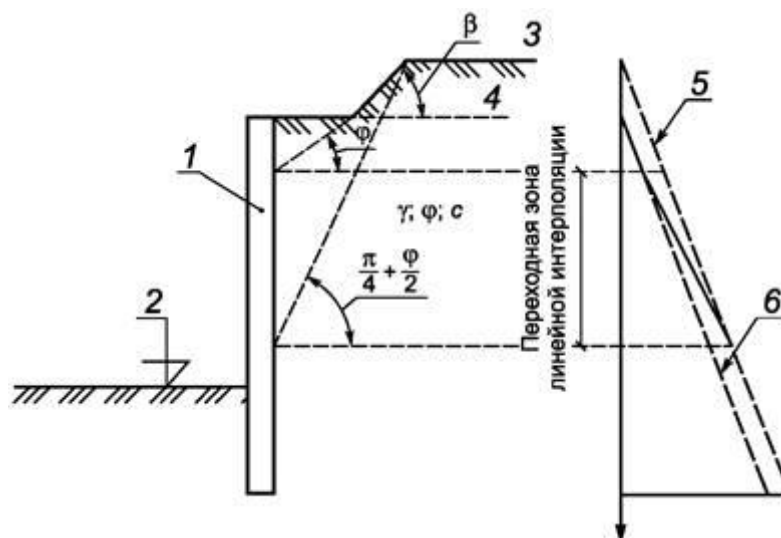
Рисунок Е.1 - Построение эпюры активного давления грунта в слоистых основаниях
