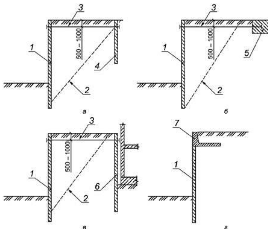
а - анкерная свая; б - анкерная плита; в - анкеровка за соседнее сооружение; г - разгрузочная плита; 1 - подпорное сооружение; 2 - призма активного давления; 3 - анкерная тяга; 4 - анкерная свая; 5 - анкерная плита; 6 - подпорное сооружение соседнего здания; 7 - разгрузочная плита
