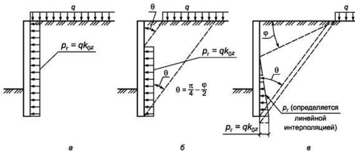
Рисунок Е.6 - Схема распределения давления p_r от полубесконечной нагрузки
