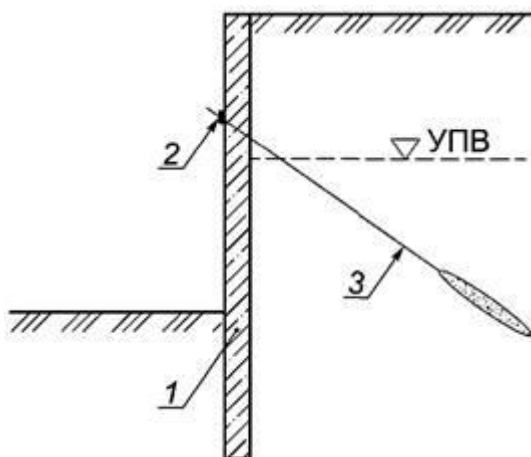
1 - подпорное сооружение; 2 - устье анкера; 3 - анкерная тяга
