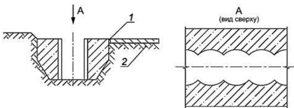
1 - деформационный шов; 2 - технологическая дорога
