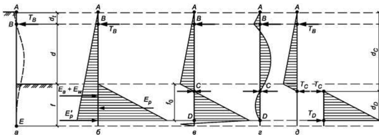
а - деформированная схема конструкции; б, в - последовательная аппроксимация активного и пассивного давления; г - эпюра изгибающих моментов в стене; д - разбиение конструкции на эквивалентные балки; d_t - глубина установки яруса крепления; d_C - глубина точки нулевого момента в стене; C - точка нулевого момента в стене; T_B - усилие в элементе крепления; T_C и T_D - усилия в условных опорах; d_D - расстояние от точки C до точки D
