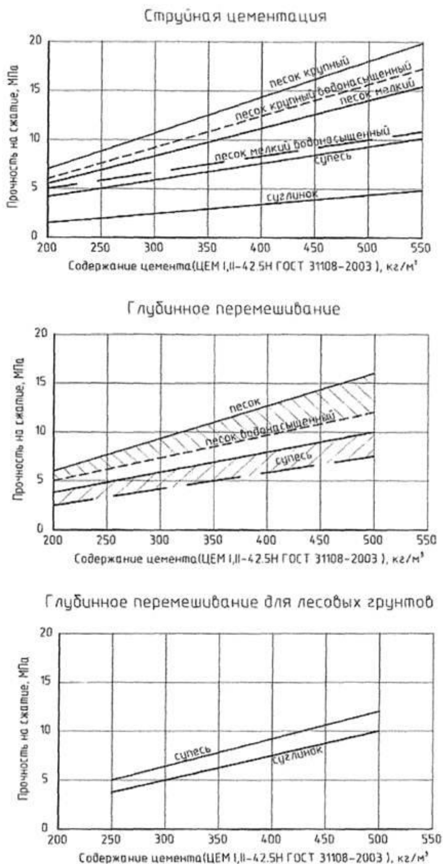
Рисунок Ф.3 - Зависимость прочности и грунтоцемента от содержания цемента в 1 м 3 ГЦЭ
